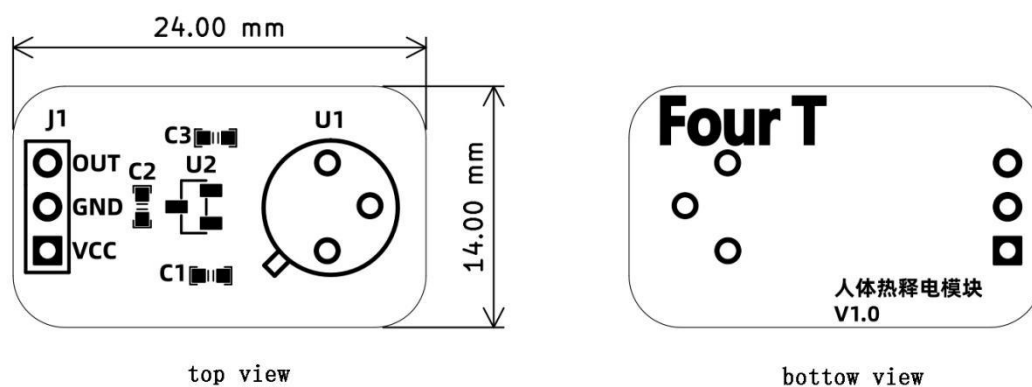
图 3.12 人体热释电模块
