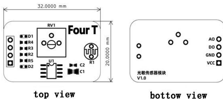
图 3.1 光敏模块
