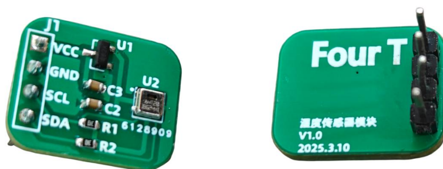
图 2.7 温湿度传感器模块
